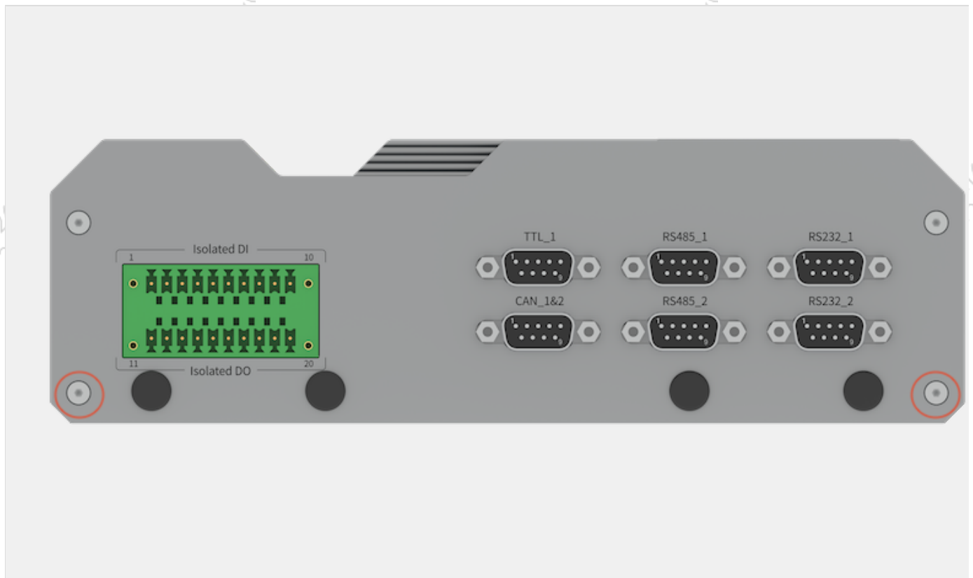
图 EVO Xavier螺丝孔位置2
