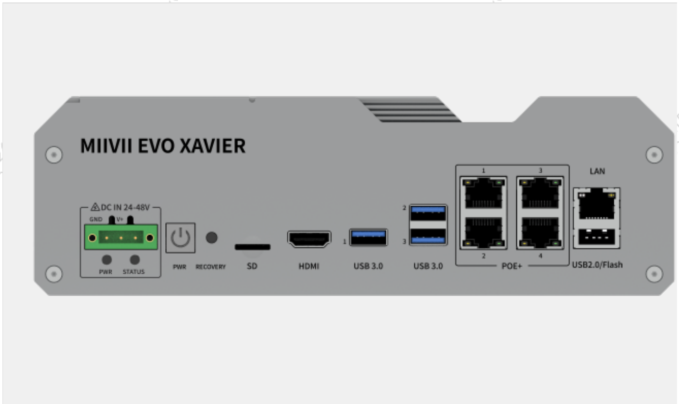
图 EVO Xavier正面接口示意图
