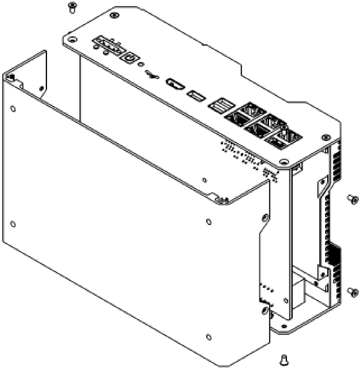
图 打开底盖
