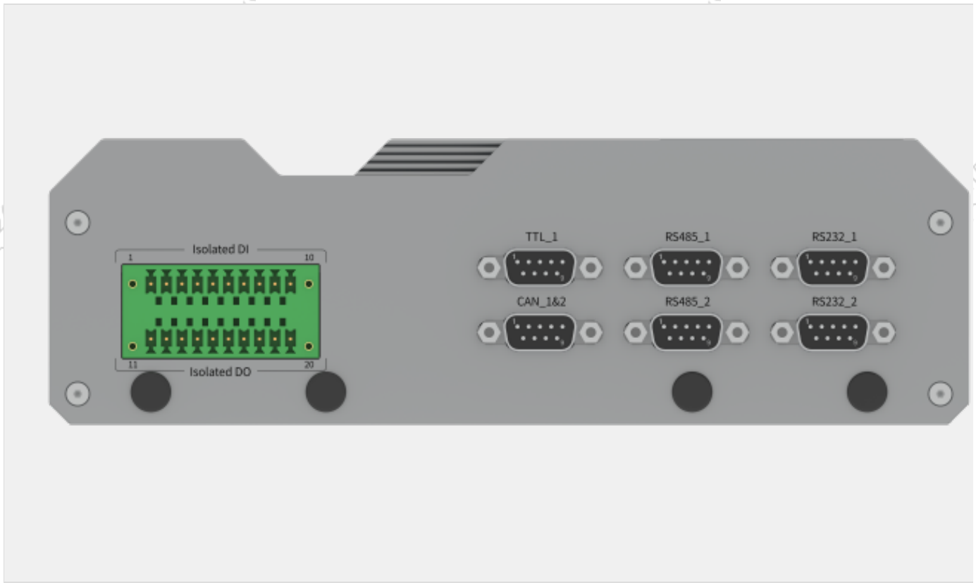
图 EVO Xavier背面接口示意图
