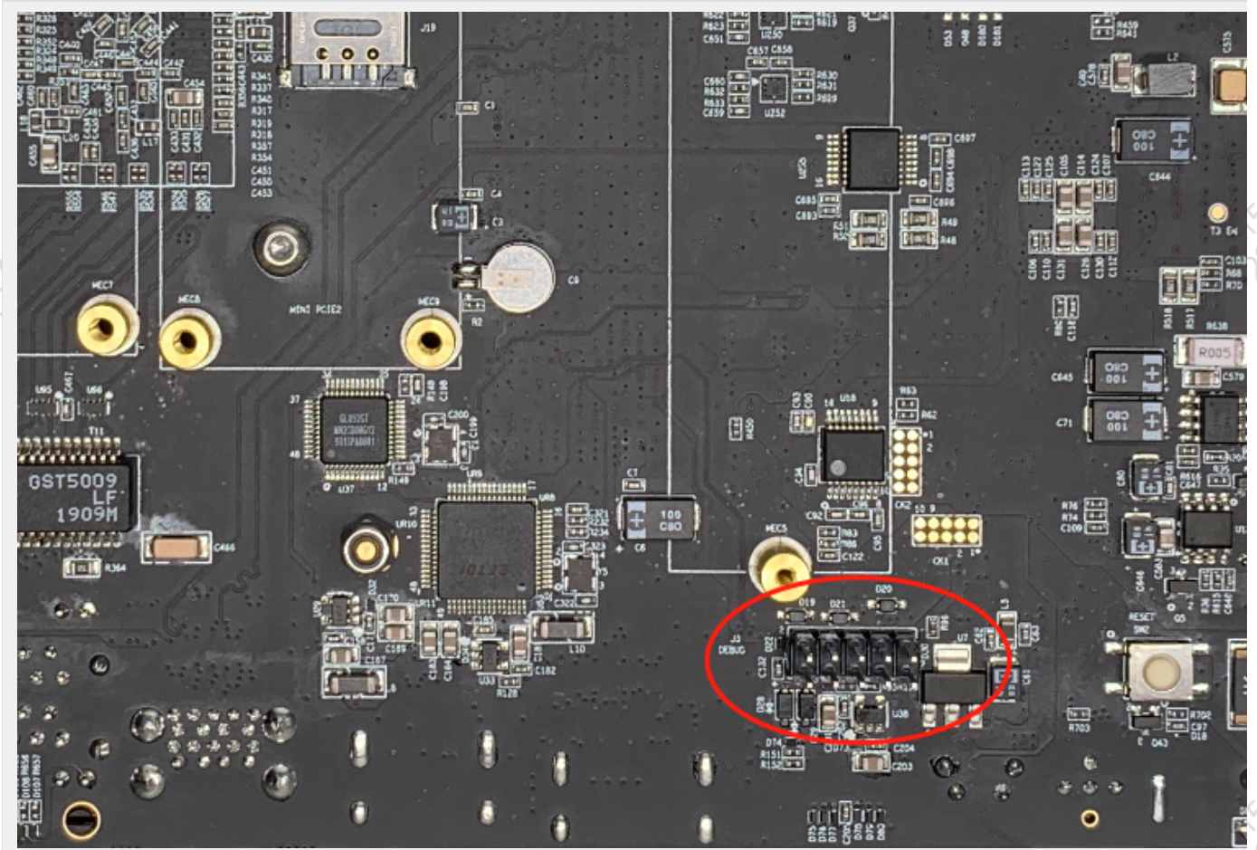
图 Debug接口位置
