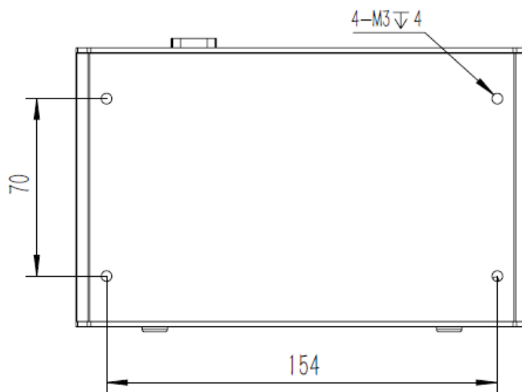
安装孔位图2 Mounting Hole(Unit:mm)
