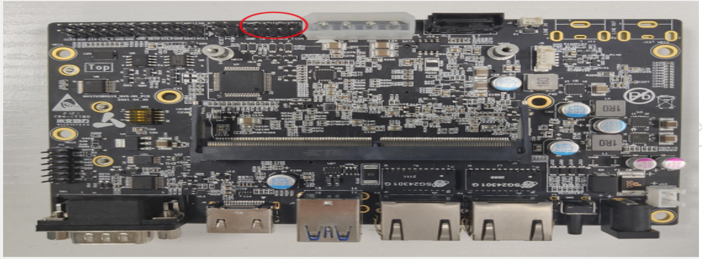
图 Debug接口位置
