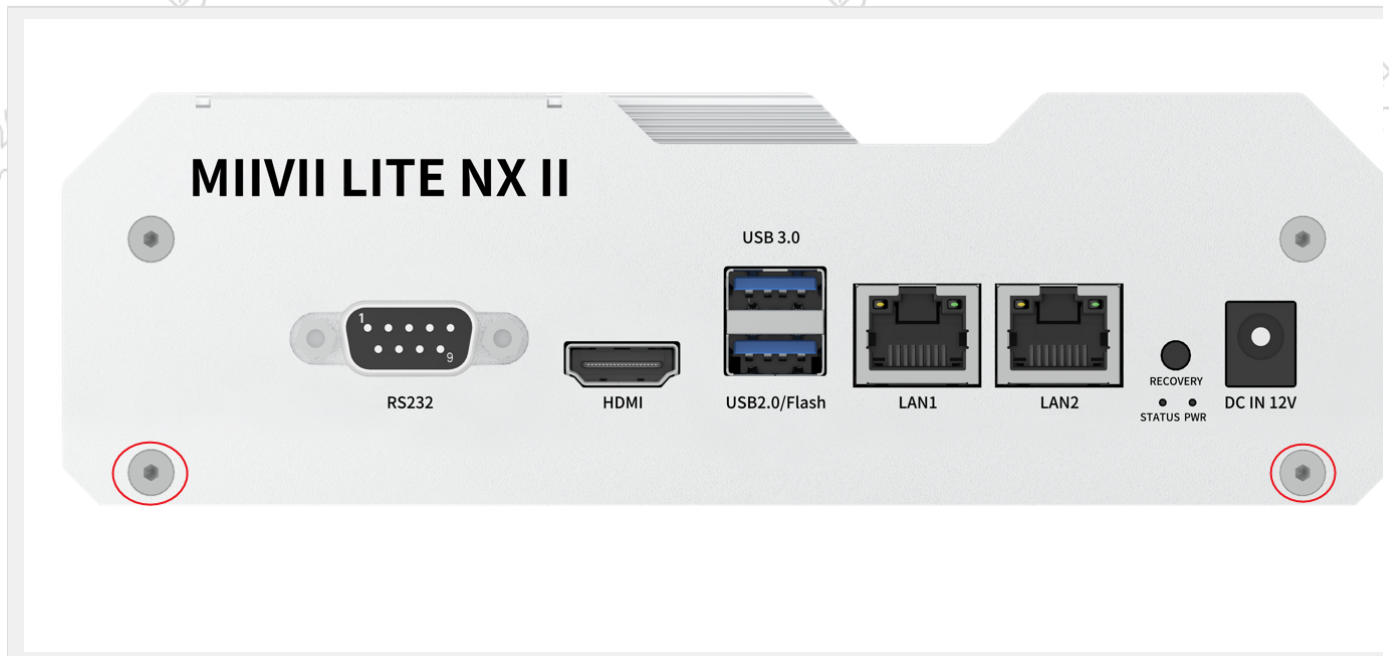
图 Lite NX II螺丝孔位置1
