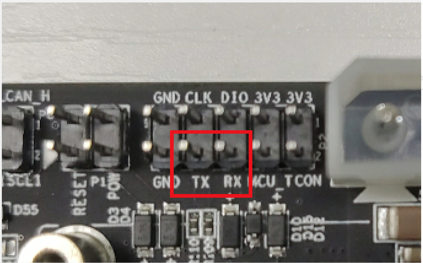
图 Debug接口序号图
