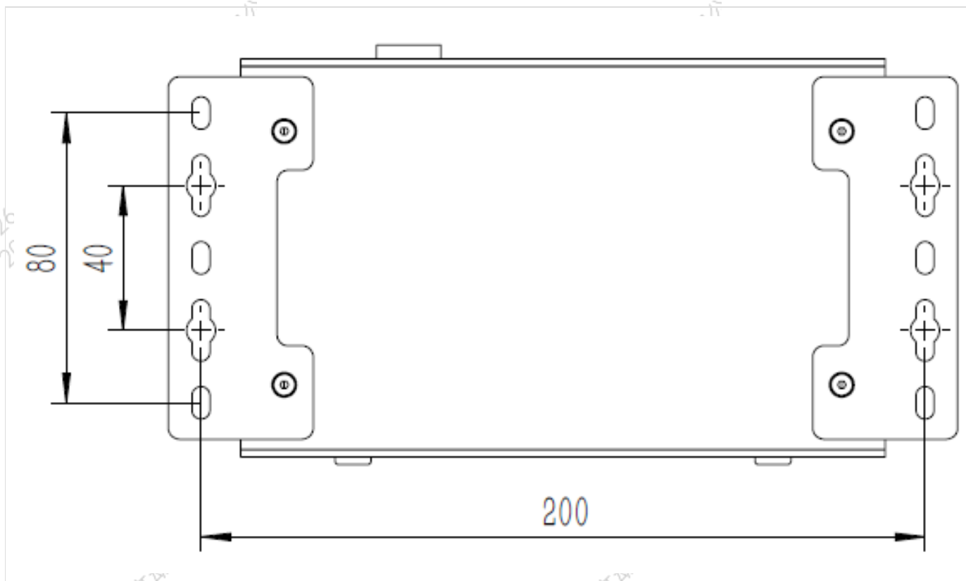
安装孔位图2 Mounting Hole(Unit:mm)
