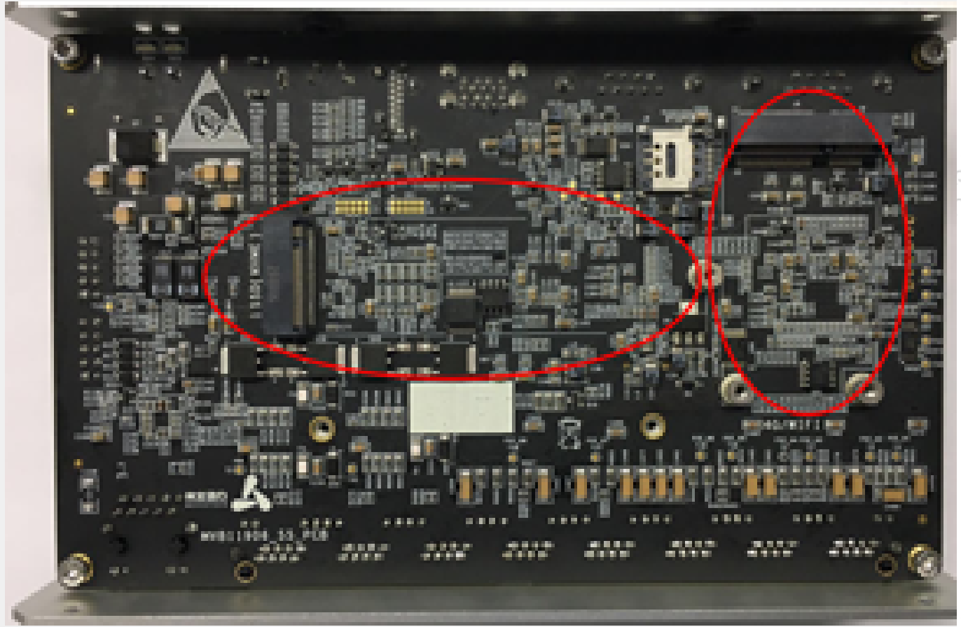
图 可扩展接口位置图
