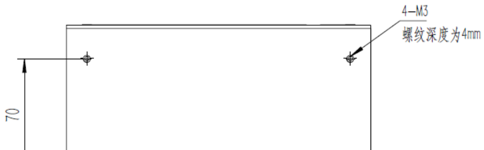
安装孔位图2 Mounting Hole(Unit:mm)
