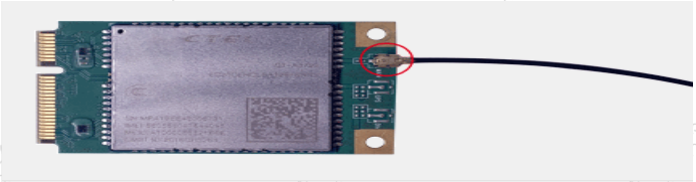
图 天线安装示意图1
