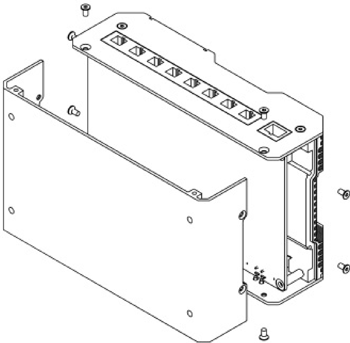
图 打开底盖
