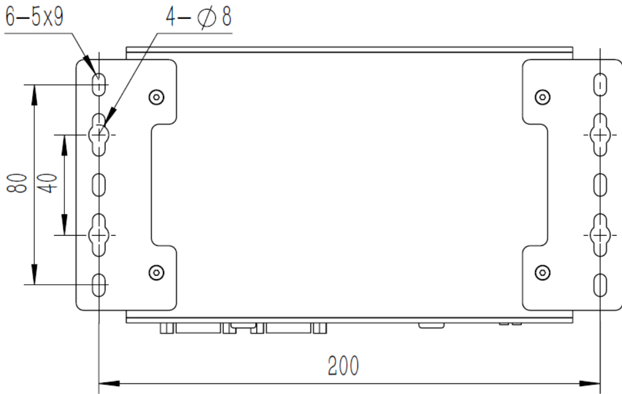
安装孔位图2 Mounting Hole(Unit:mm)
