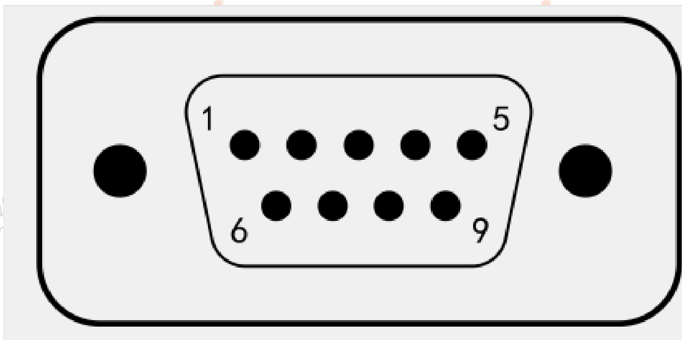
图 RS232接口序号图
