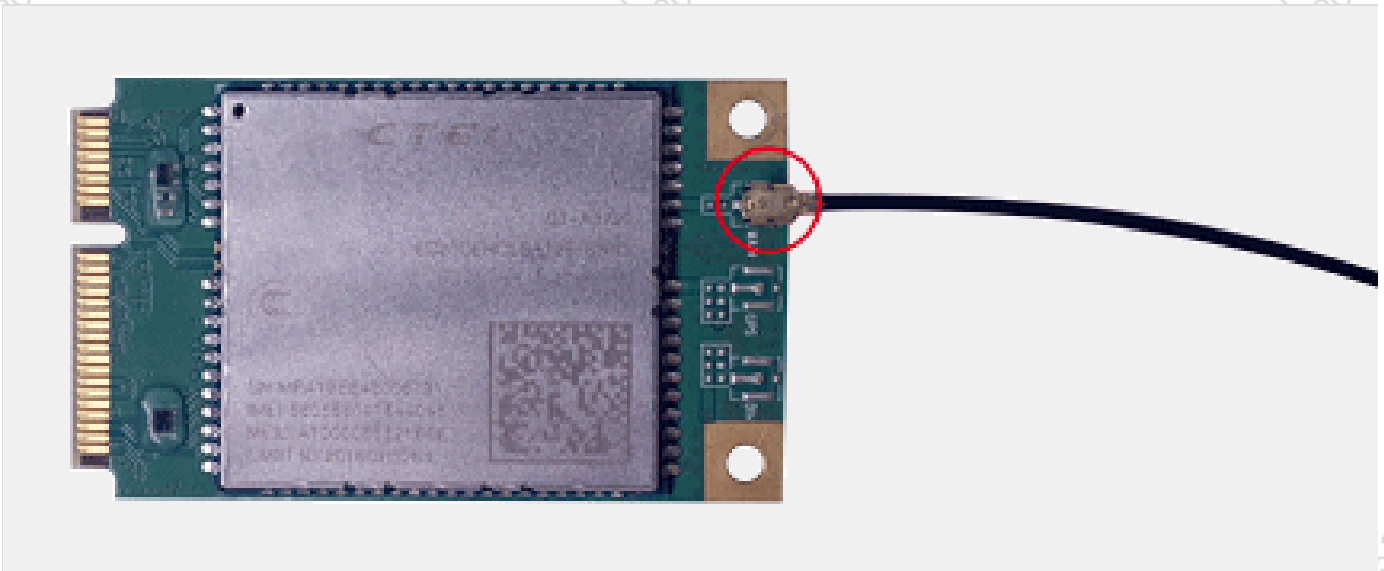
图 天线安装示意图1
