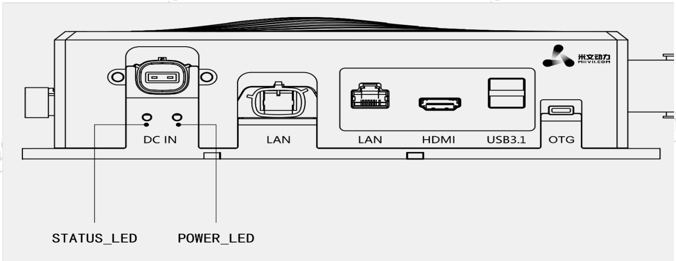
图 Apex Xavier正面接口示意图
