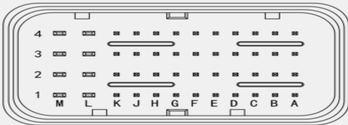
图 EXPANSION PORT 接口序号图
