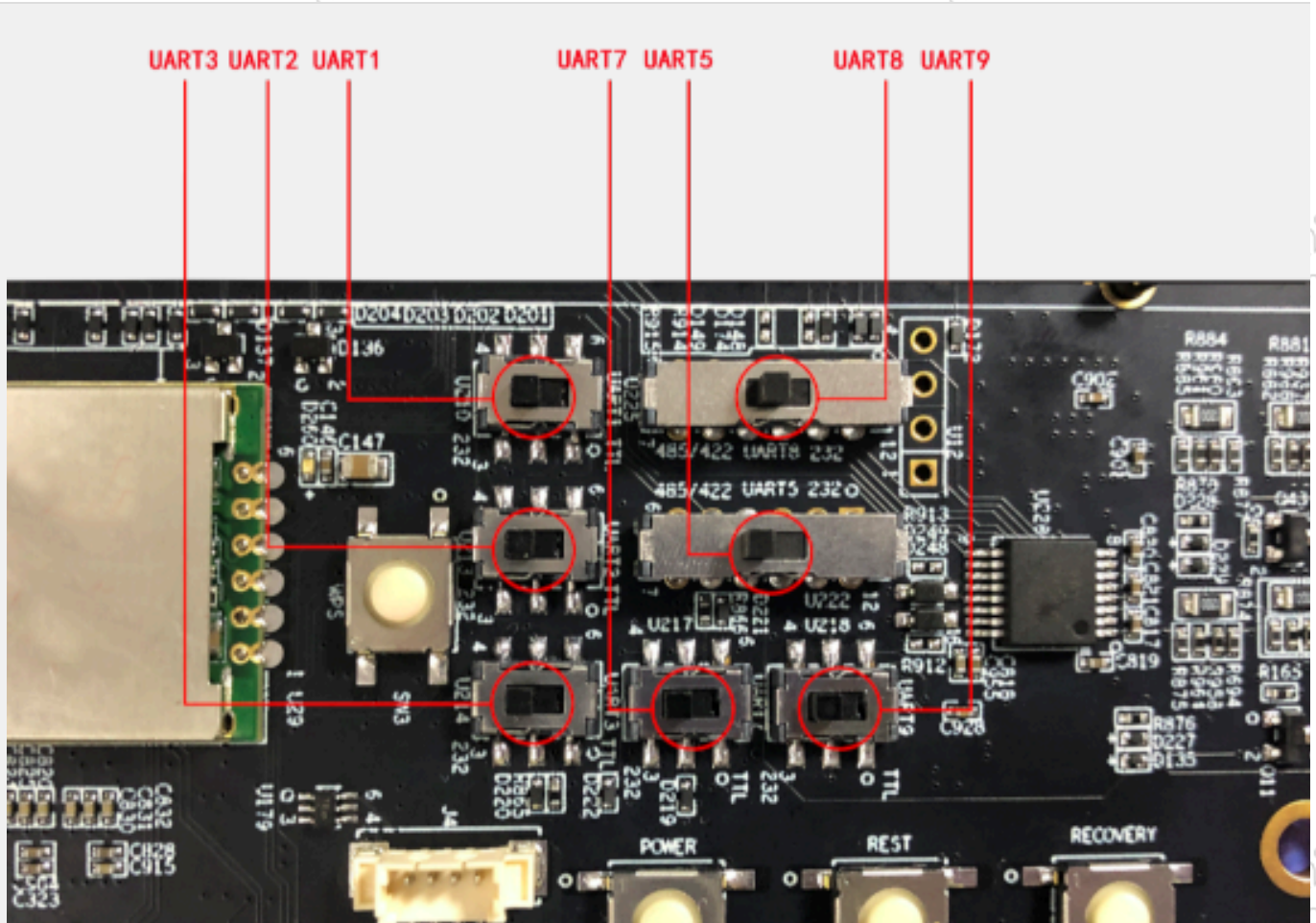
图 拨码开关示意图
