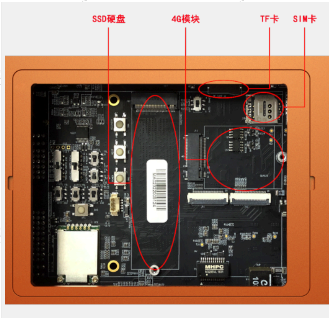
图 SSD硬盘 4G模块 TF卡 SIM卡安装位置图
