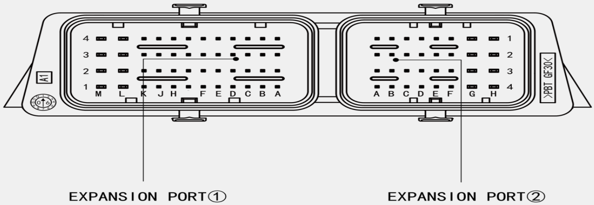
图 多功能接口图
