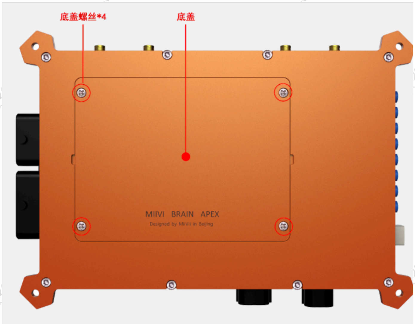
图 Apex Xavier底盖及螺丝位置
