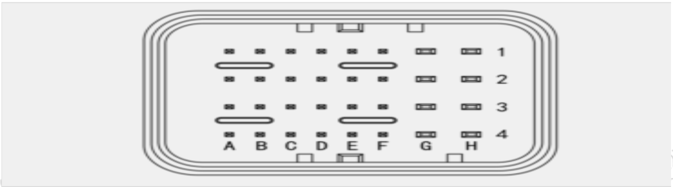
图 EXPANSION PORT接口序号图
