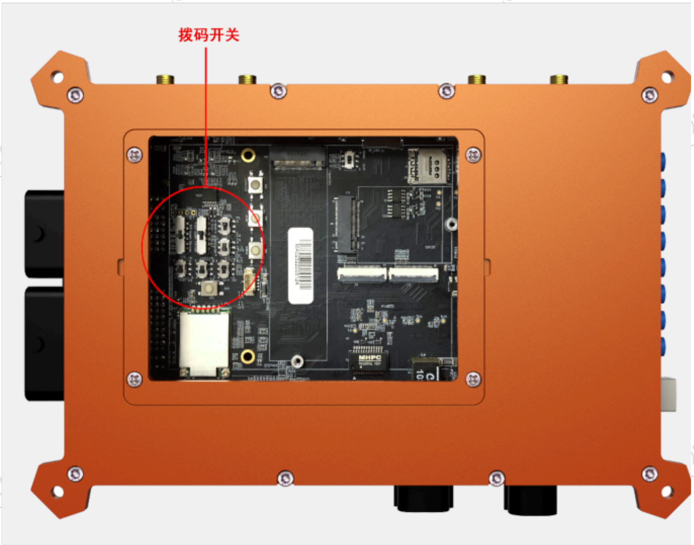
图 拨码开关实物位置图
