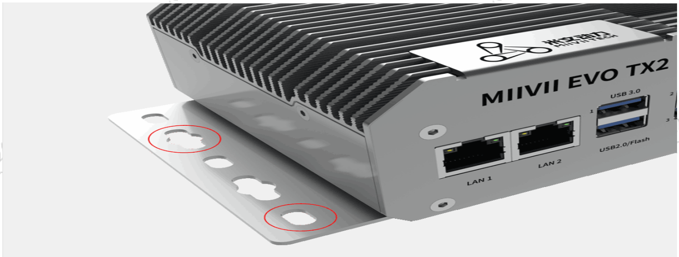
图 EVO TX2固定示意图
