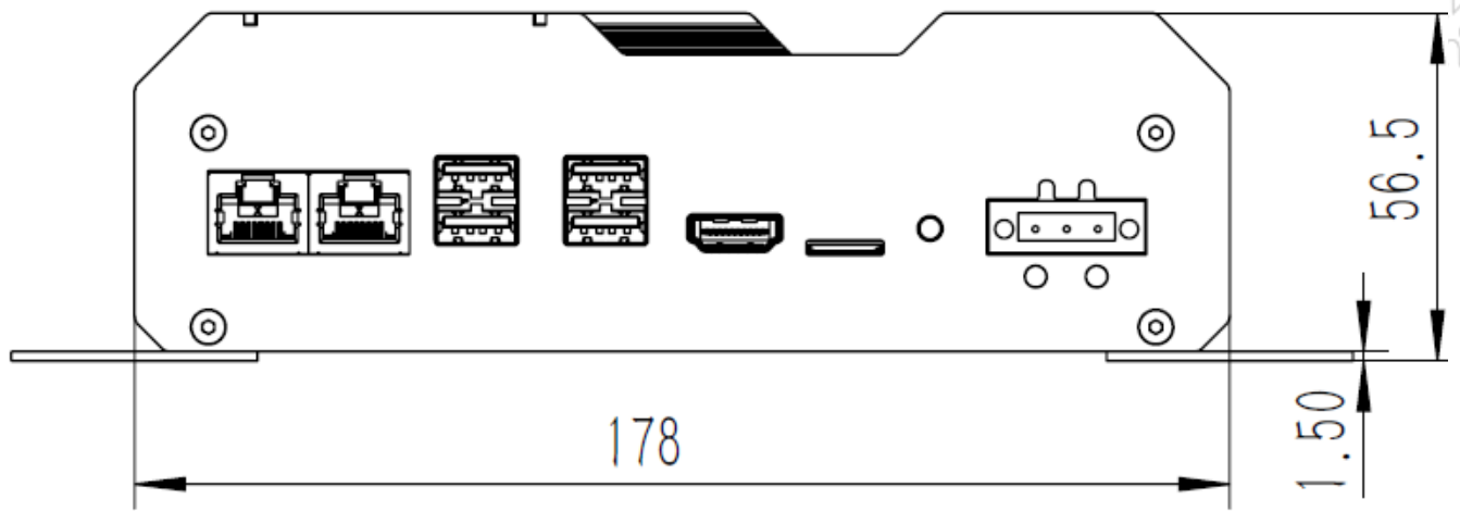
左视图 Left view(Unit:mm)
