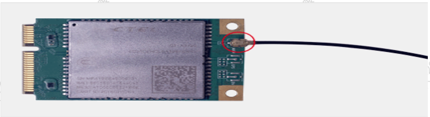
图 天线安装示意图
