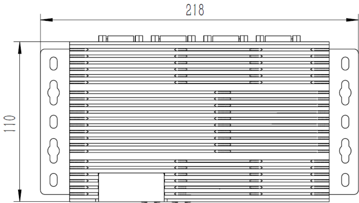
主视图 Front view(Unit:mm)
